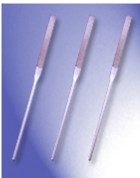
PF-70: 140L x 40~50T x Ø3.0B Körnung : #150, #200, #400
